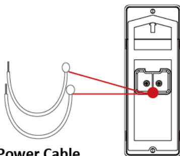
Obrázek 2-3. Připojení dodaných napájecích kabelů
